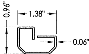
35 ASTRAGAL
